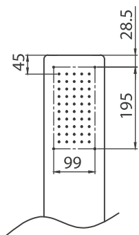
פאנל אחורי
